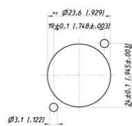
Frontplatten-Ausschnitt (von hinten)
